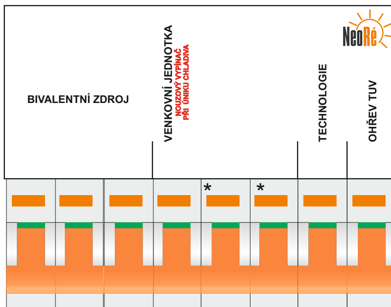
Jisticí prvky tepelného čerpadla -tří fázové provedení
